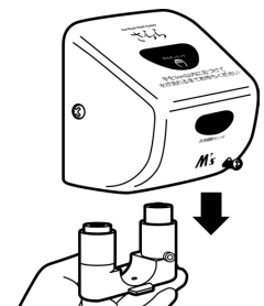
電池ケースが下方向へ外れる
