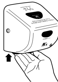
電池ケースを上へ押すと固定金具が外れる
