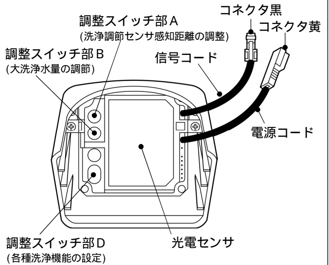
【センサケース内側】 裏ボタンを外したとき
