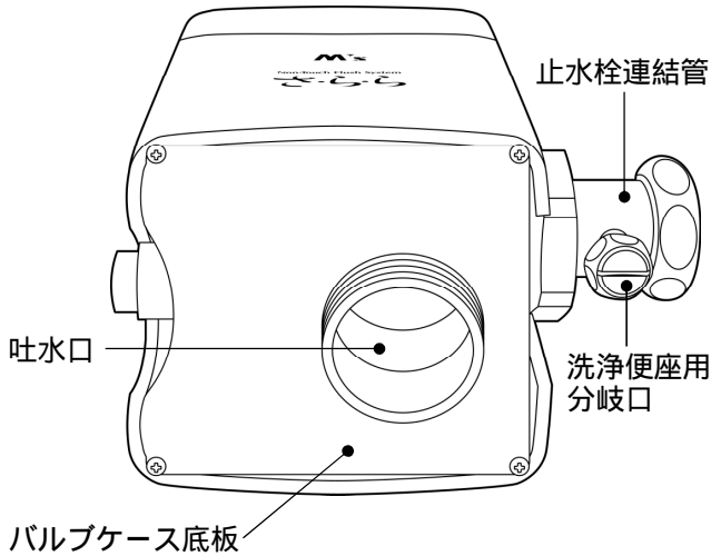
【バルブ部底部】
