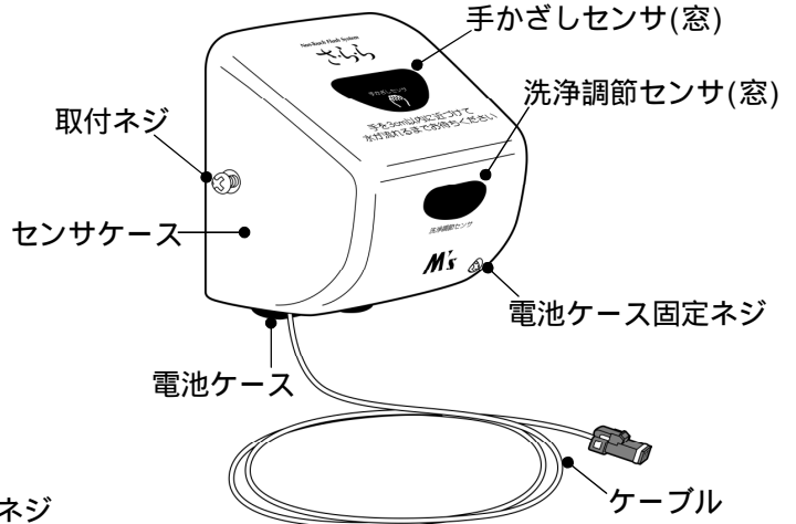
【センサ部前から】
