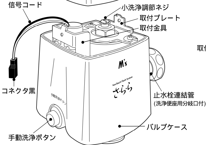
【センサケース裏から】
